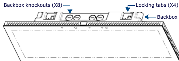
FIG. 3 MXD-1900L-PAN (LANDSCAPE)
